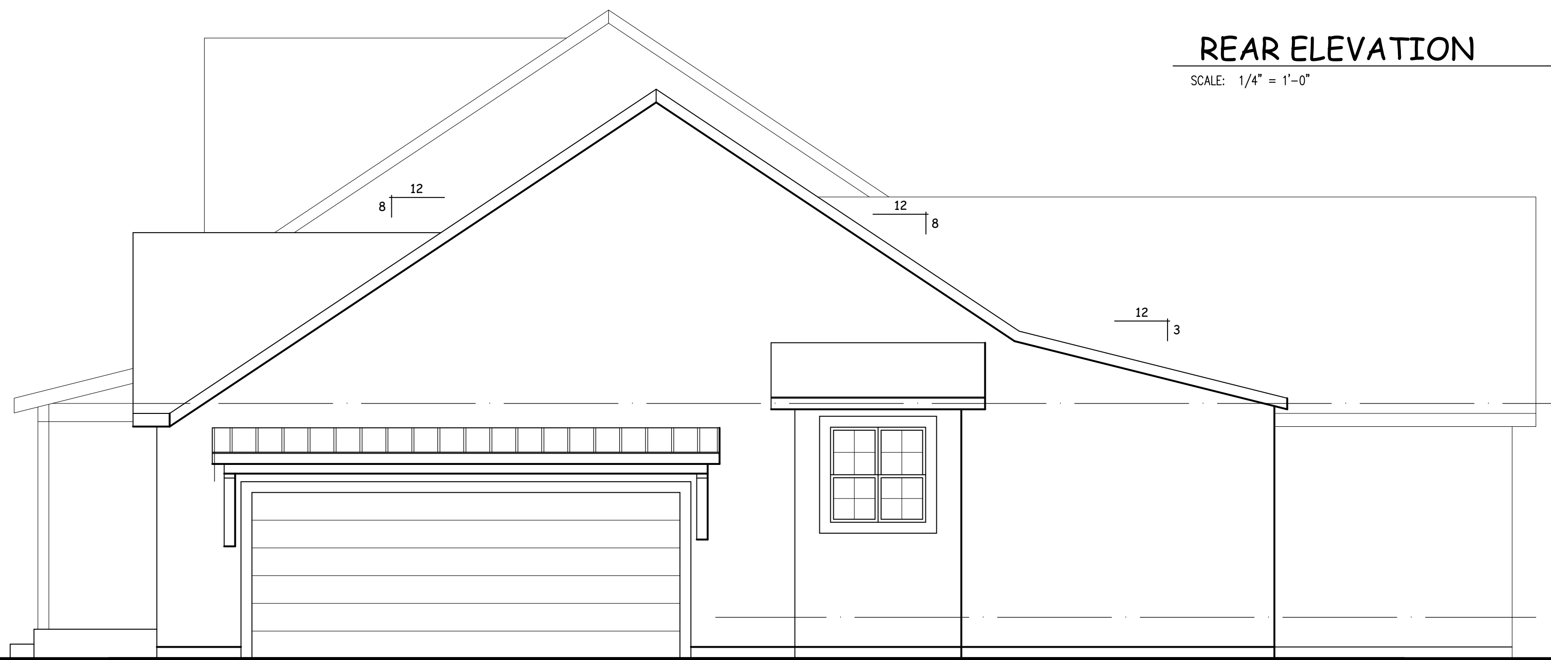
RIGHT ELEVATION
